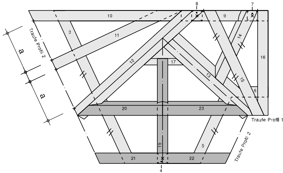
Grundriss mit Schwellenlage
