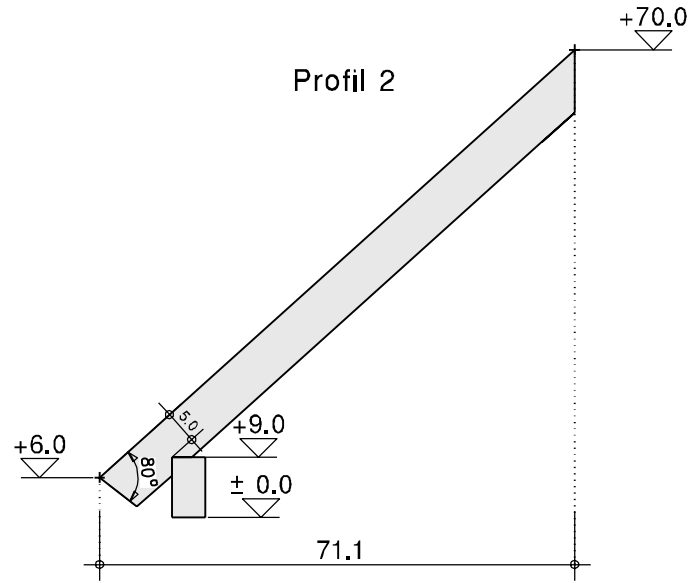
Holzliste Modul 1
