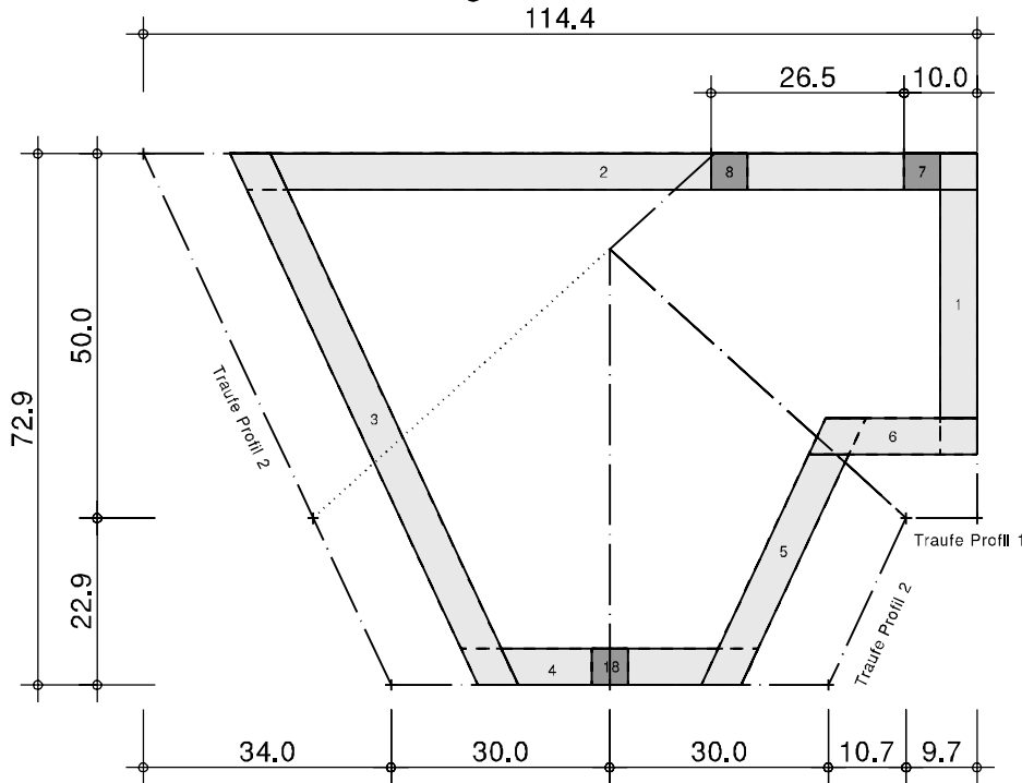
Grundriss mit Schwellenlage
