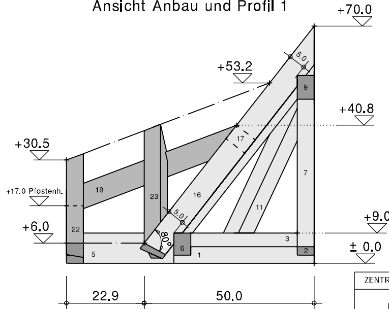
Ansicht Anbau und Profil 1
