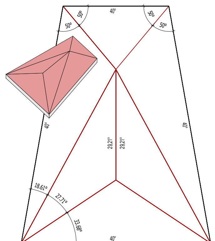
waagerechter First, HD-Flächen trianguliert, nur ebene Dachflächen, zusätzliche Grate
