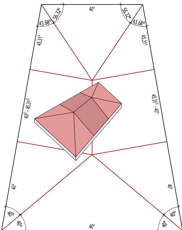
waagerechter First, gerade Grate, HD zwischen Anfallpunkten windschief
