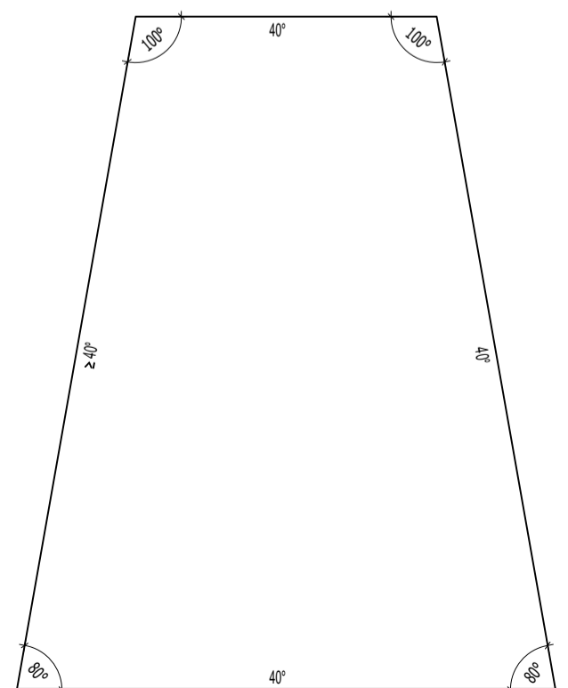
waagerechter First, HD-Flächen trianguliert, nur ebene Dachflächen, zusätzliche Grate
